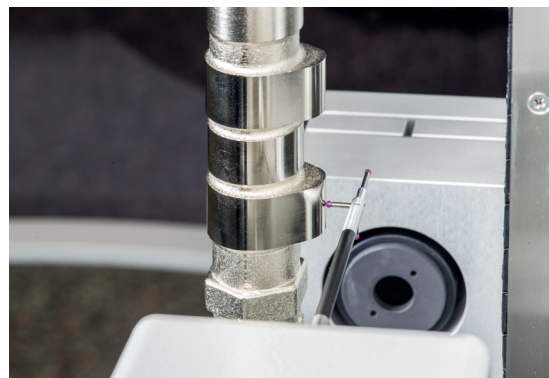
Nockenform messen
